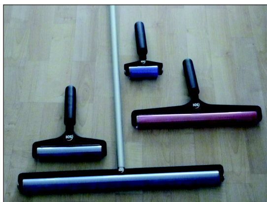
Standard - Handreinigungsroller in verschiedenen Größen und Klebeausführungen
