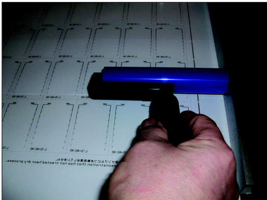
Handreinigungsroller mit einseitiger Rollenführung zum kanten- bzw. ecknahen Reinigen der Oberflächen (Breite 150 mm)
