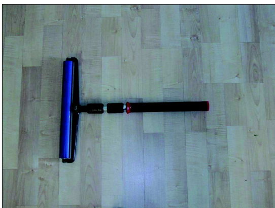
Handreinigungsroller mit verstellbarem Teleskop-Griff (Gesamtlänge 450 - 835 cm)
